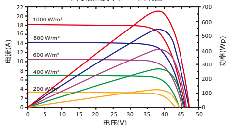
RSM132-8-680BNDG 不同辐照度下, I-V 曲线图
